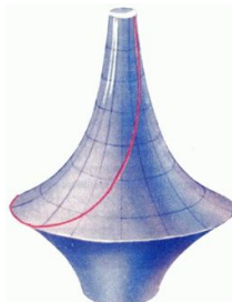
Рис.6. Псевдосфера Бельтрами
